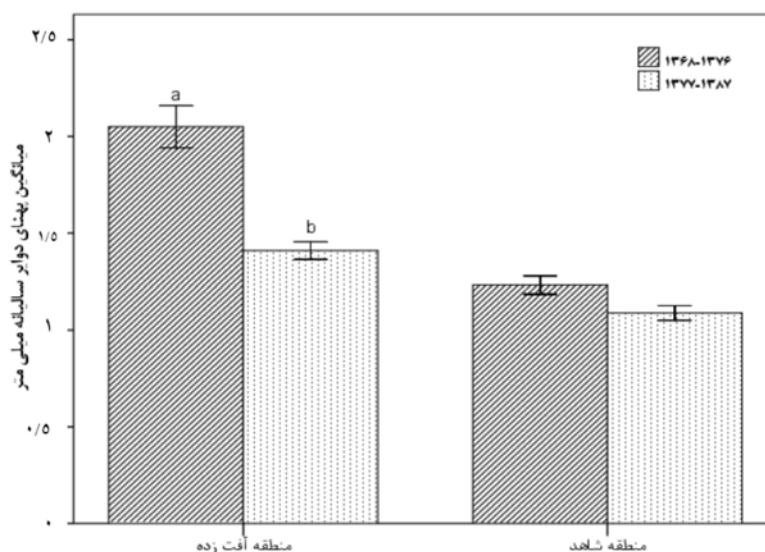
شکل ۲- میانگین پهنای دواير سالیانه بلوط و بول Q. libani در مناطق آفت‌زده و شاهد در دو دوره زمانی قبل (۱۳۷۶-۱۳۷۸) و بعد از شیوع آفت (۱۳۷۷-۱۳۸۷)
