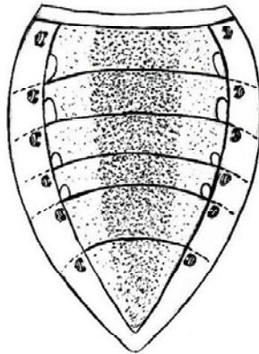
شکل ۲- نمای سطح زیری شکم در سن Coranus subaptreus De Geer
